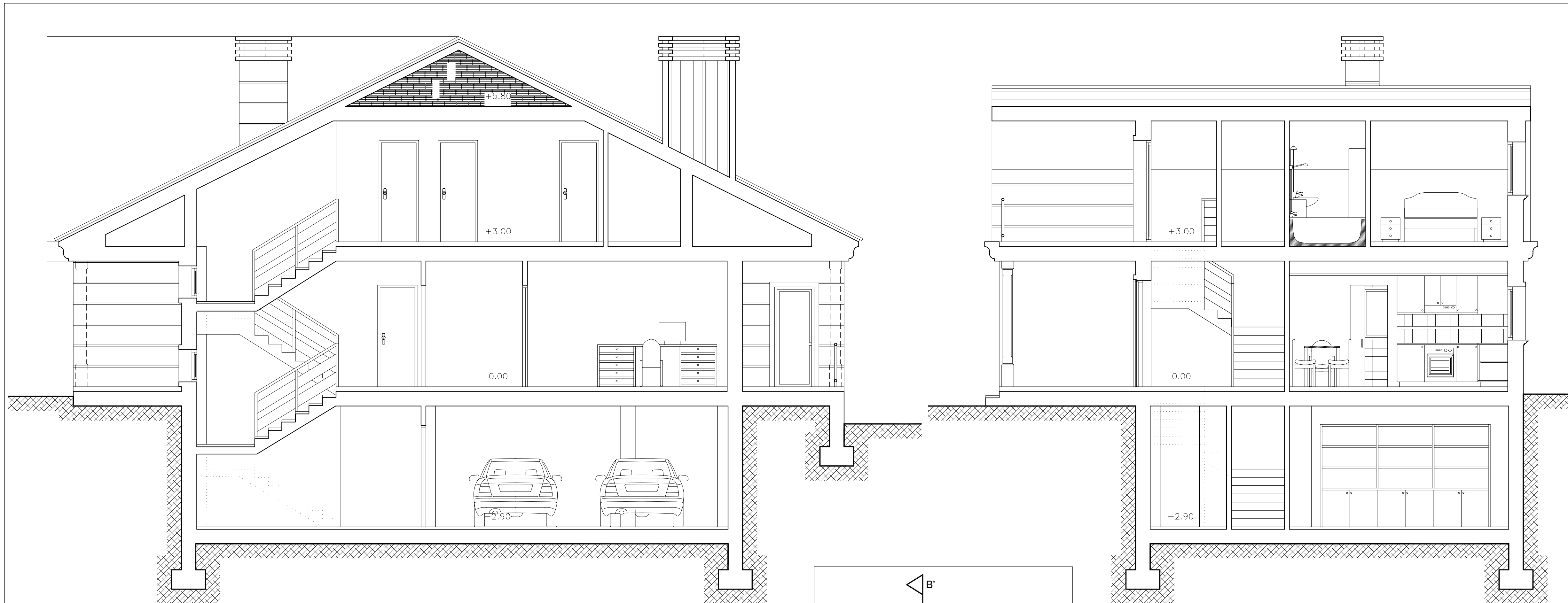
SECCIÓN A-A'
